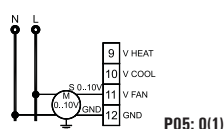
Fig. 13a. Collegamento di un ventilatore proporzionale con motore elettronico (EC motor) con ingresso 0..10V. Connection of a proportional fan with an EC motor with 0..10V input.
