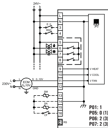
Fig. 9: Schema di collegamento per pilotaggio di due attuatori on/off a 24V ~ per impianto a 4 tubi e pilotaggio proporzionale del ventilatore. Wiring diagram for 2 on/off 24V ~ actuators in 4 pipes system and proportional fan drive.
