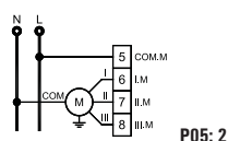
Fig. 13b. Collegamento di un ventilatore con motore a tre velocità. Connection of a fan with a three speeds motor.
