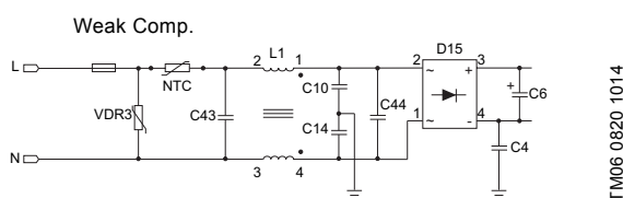
Fig. 42 NTC
