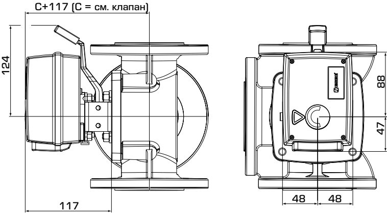
Установочные размеры для приводов серии CRA120 со смешивающими клапанами ESBE серий MG, G, F, T/TM, H/HG и BIV
