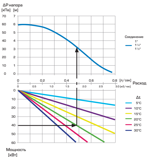
LTC260 – доступное давление насоса
