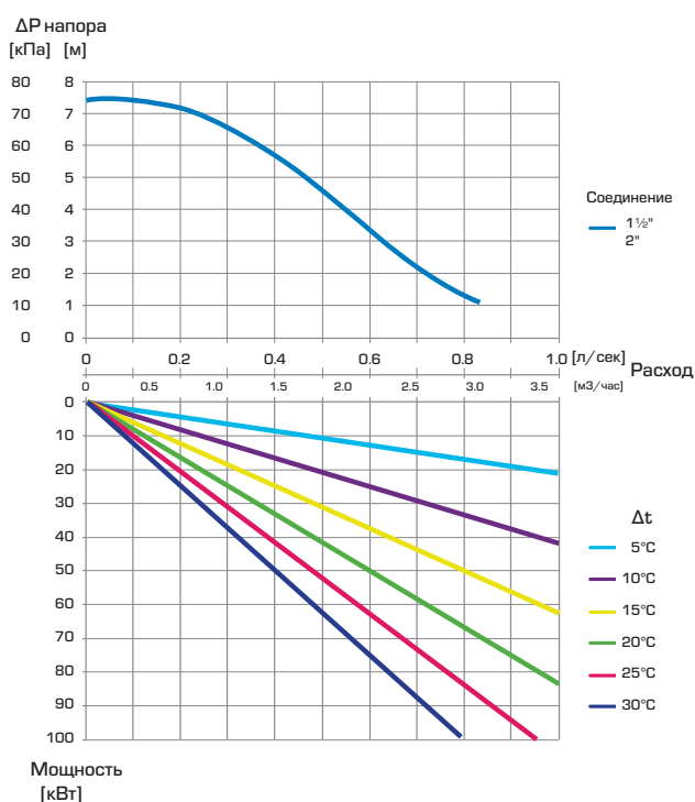
LTC270 – доступное давление насоса
